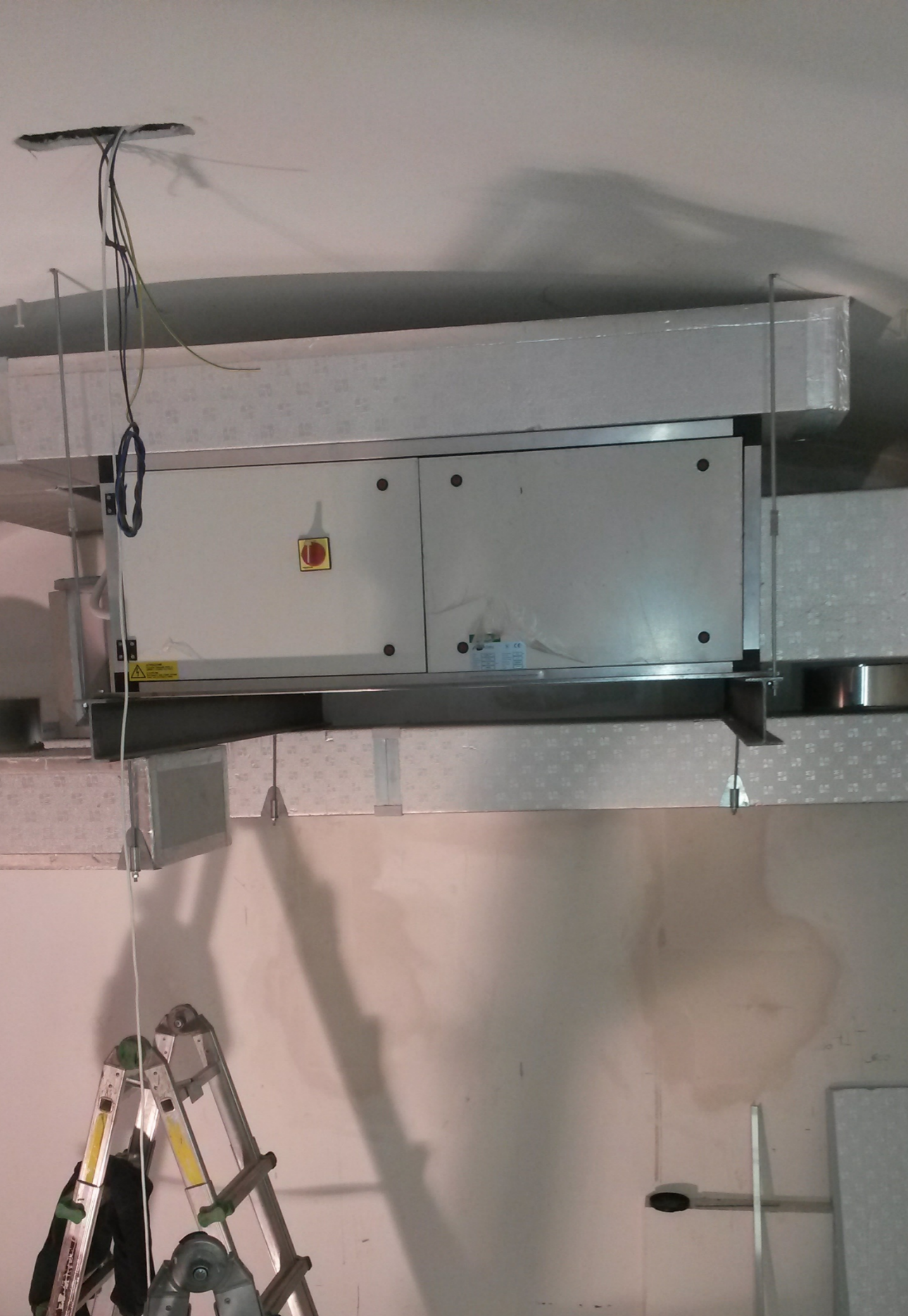
Impianto di trattamento aria e climatizzazione estiva e invernale
